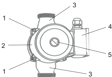
Рис. 1. Конструкция насоса.
